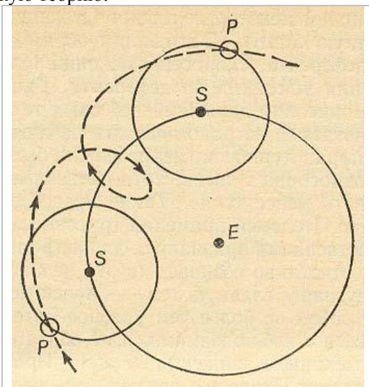
Рис. 1.5. Эпицикл и деферент
