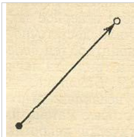
Рис. 4.5. Вектор
