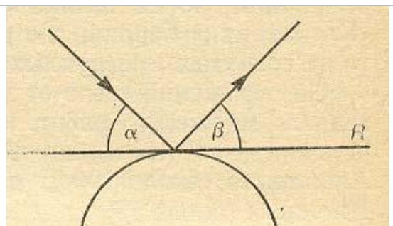
Рис. 1.7. Отражение от выпуклого зеркала
