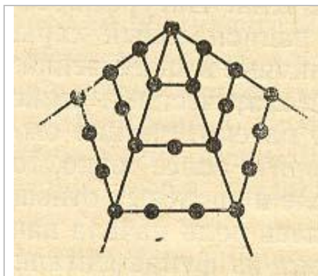
Рис. 1.3. Пятиугольные числа
