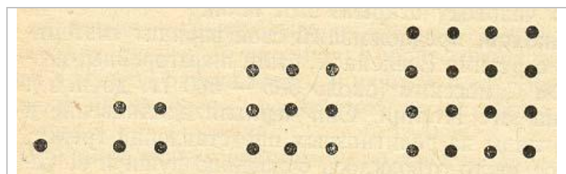
Рис. 1.2. Квадратные числа
