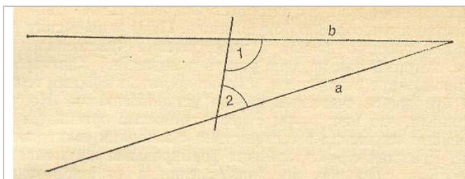
Рис. 4.1. Пятый постулат Евклида
