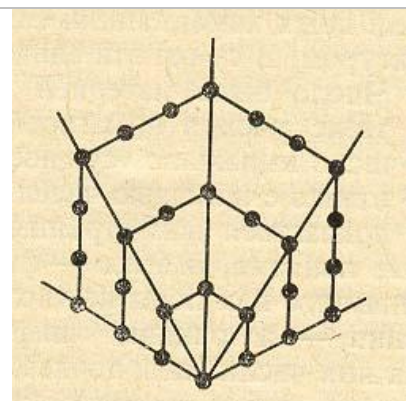
Рис. 1.4. Шестиугольные числа
