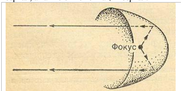
Рис. 1.8. Отражение от параболического зеркала.
