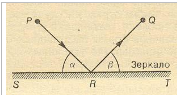
Рис. 1.6. Отражение от плоского зеркала
