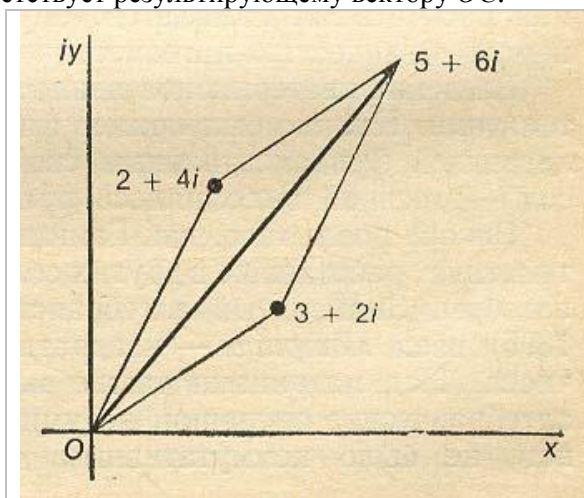
Рис. 4.7. Сложение комплексных чисел по правилу параллелограмма
