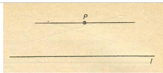
Рис. 4.2. Вариант аксиомы о параллельных, предложенный Джоном Плейфером
