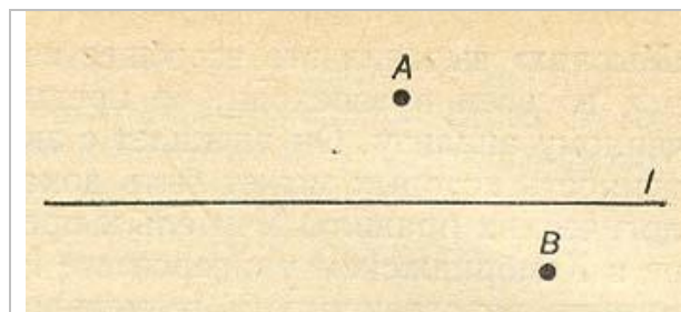
Рис. 5.1. Аксиома, которую не сформулировал Евклид
