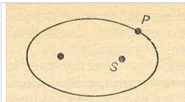
Рис. 2.1. Первый закон Кеплера. Планеты движутся по эллипсам, в одном из фокусов которого находится Солнце
