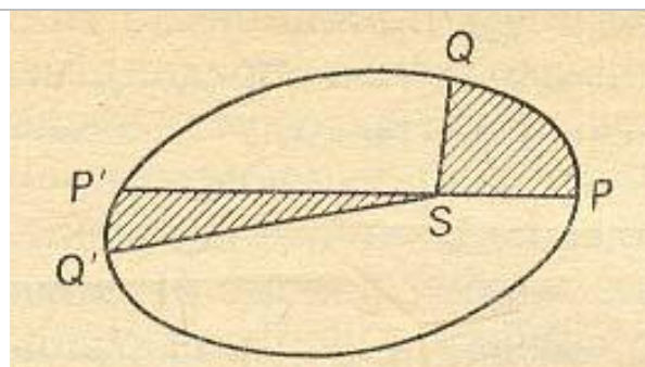
Рис. 2.2. Второй закон Кеплера: если дуги PQ и P'Q' орбиты планеты проходят за одно и то же время, то площади секторов PSQ и P'SQ' равны
