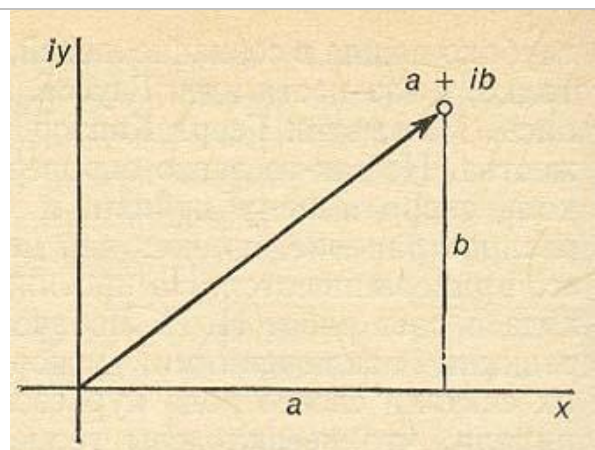
Рис. 4.6. Геометрическое представление комплексных чисел
